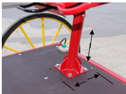
Réglage de la potence du siège en hauteur ainsi que d'avant en arrière sur le plancher, Le siège meneur se règle également d'avant en arrière
